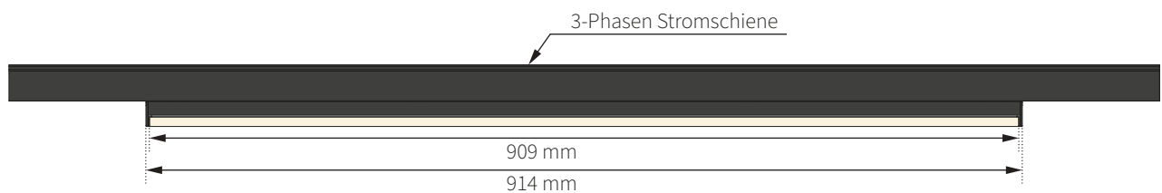
Maßstab 1:1 scale 1:1
